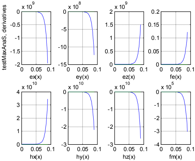
Fig. 9.6.1b, modeFig=1, mode=2, modeZ=2.
