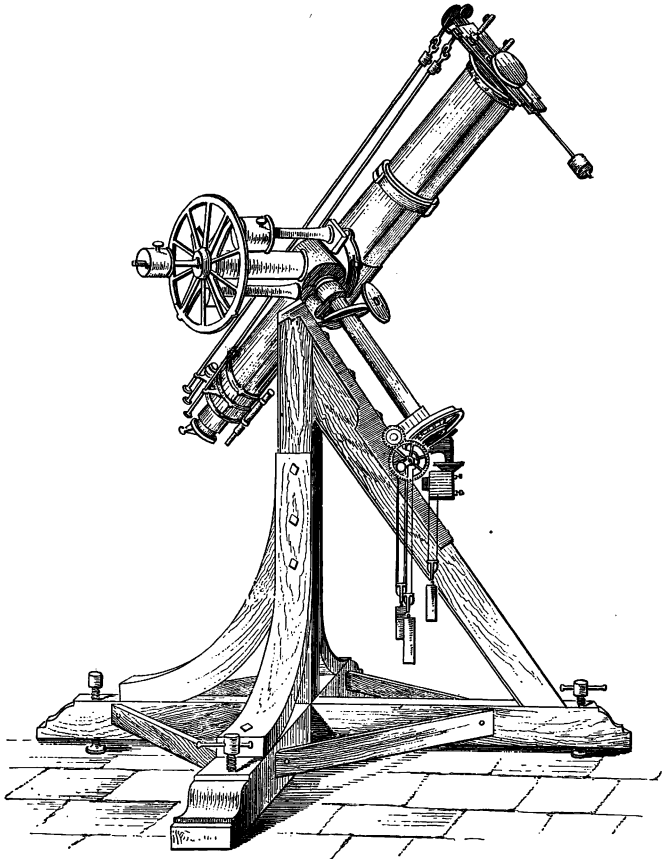
FIG. 92.—Heliometer.
