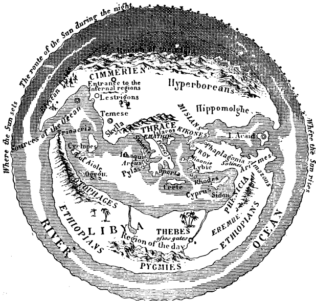
FIG. 4.—Homeric Cosmogony.
