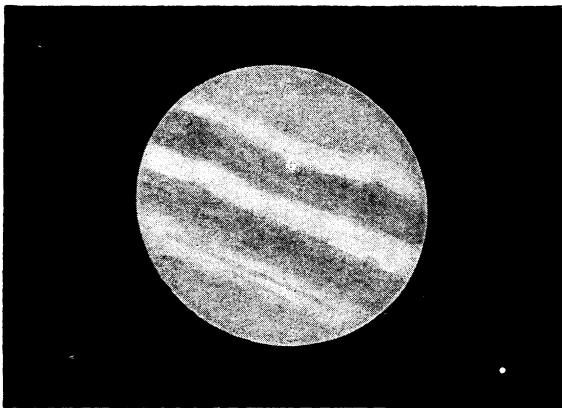
FIG. 72.—Jupiter.
