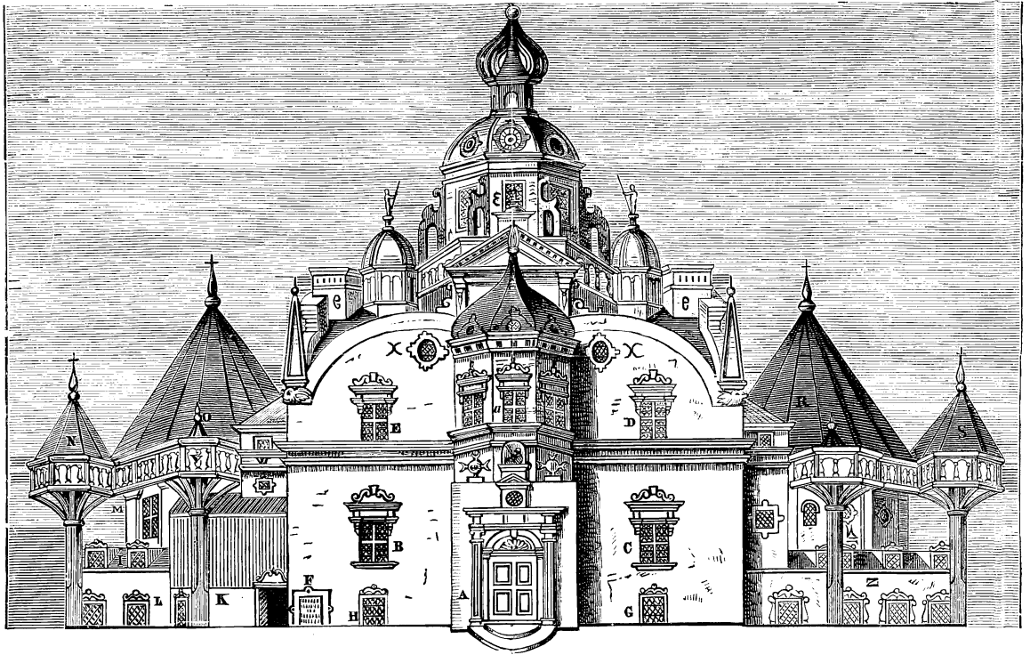
FIG. 20.—Uraniburg.
