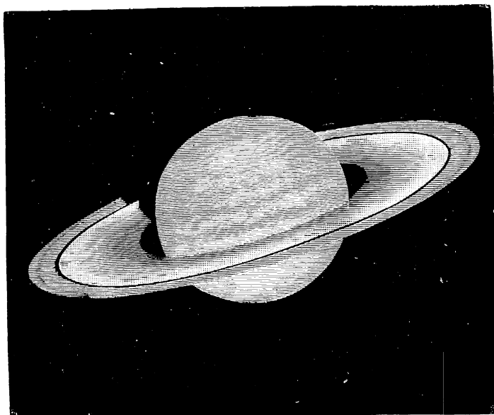
FIG. 81.—Saturn.
