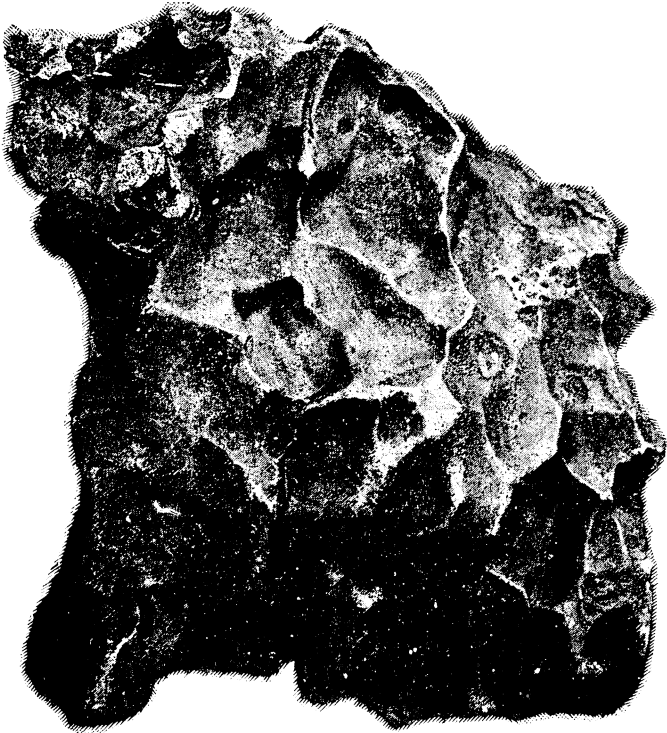
FIG. 95.—Meteorite.
