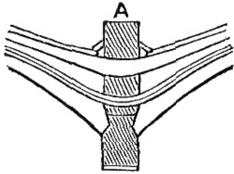
A, Keelson.
